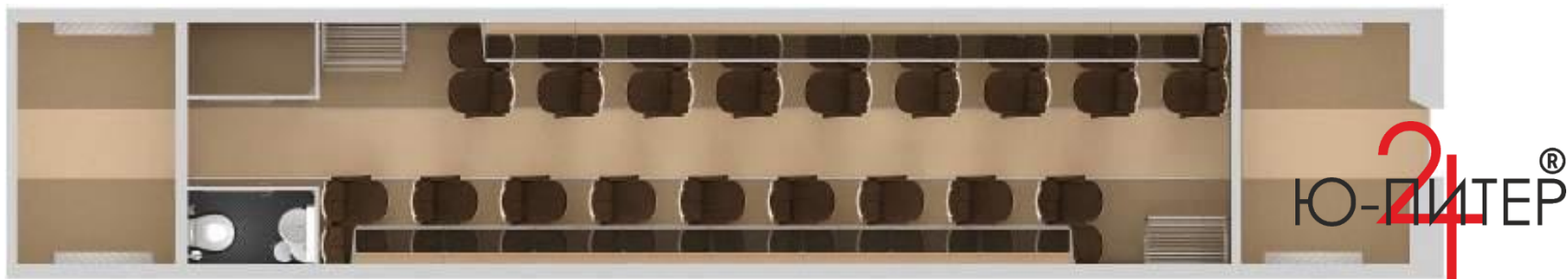
Рис.3. План головного вагона
